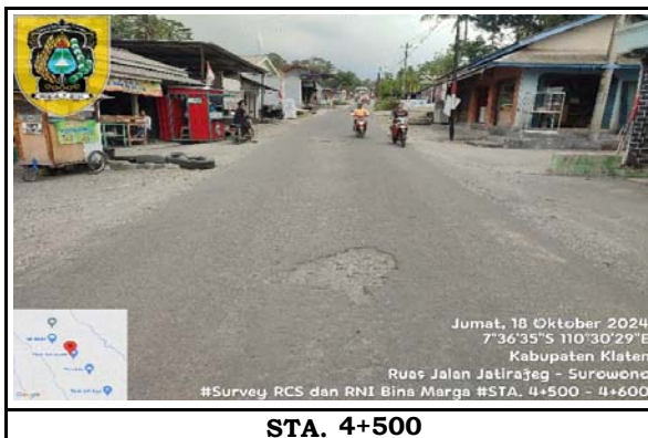
STA. 4+500
