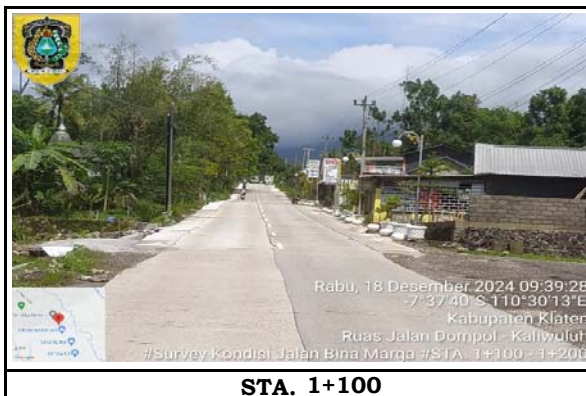
STA. 1+100
