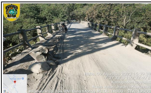
STA. 1+810
