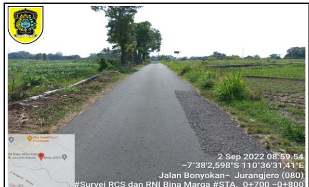
STA. 0+700
