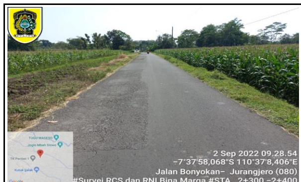
STA. 2+300
