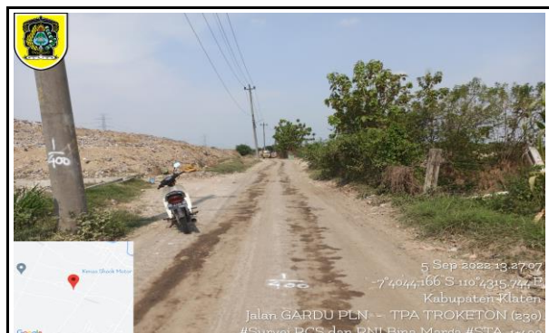
STA. 1+400
