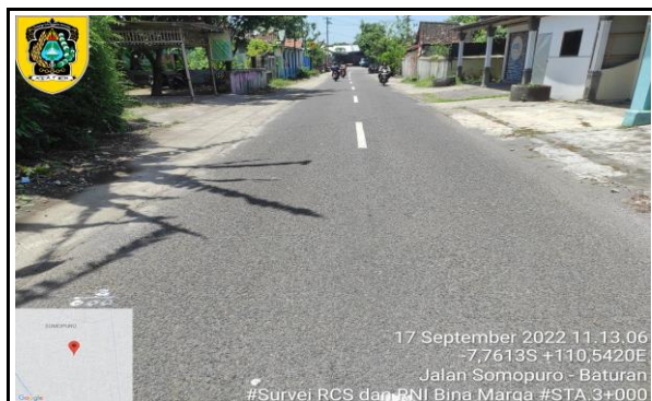
STA. 3+000
