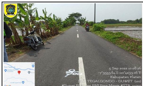
STA. 0+700
