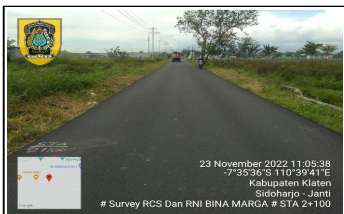
STA. 2+100
